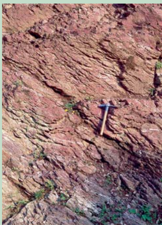
Radiolarit a bánya-hegyi szelvényben (B. Cs.)
