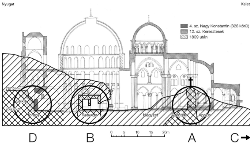
2. ábra. A Szent Sír-templom hosszmetete (Kroll, G. 1985 szerint) a Jézus korabeli sziklafelszín rekonstrukciójával és a napjainkig fennmaradt szálkőzet-részletekkel.
