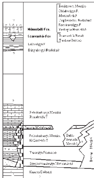
A déli-bükki szerkezeti egység földtani képződményeit bemutató rétegszlop
